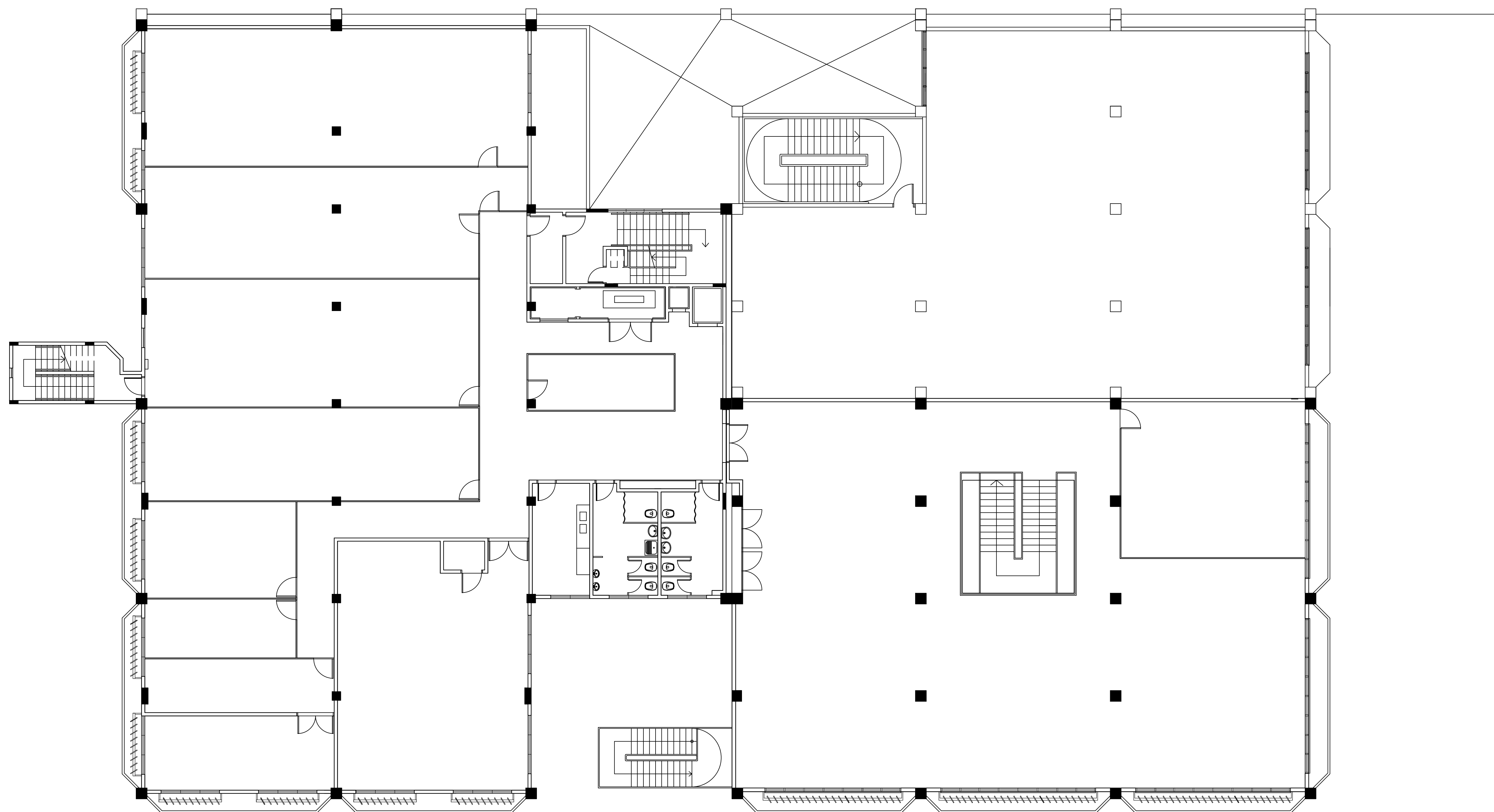
PLANTA DO 2º PAVIMENTO - NÍVEL 744,10 ESCALA 1:100
